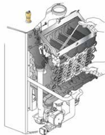
Für Reinigungsarbeiten ist der Wärmetauscher aus Aluminium/Silizium-Sandguss einfach und vollständig zugänglich.
