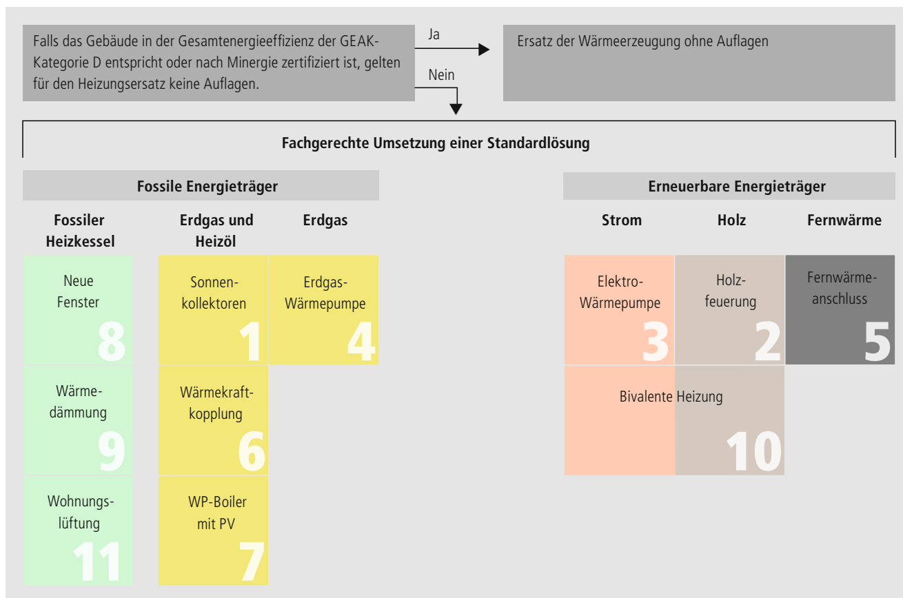
Fünf Energieträger für elf Standardlösungen: die MuKEn-Vorgaben für den Ersatz der Wärmeerzeugung
